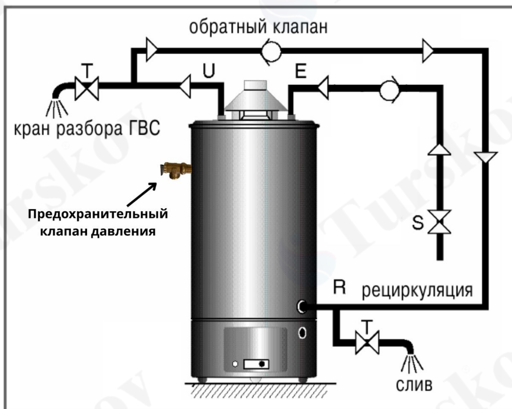
Схема 3. Подключение к сети водоснабжения.
